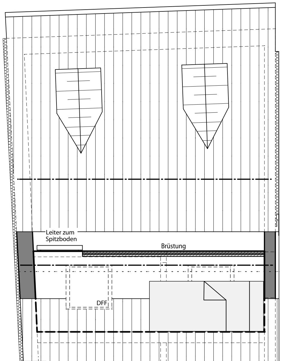
Schlafgalerie
