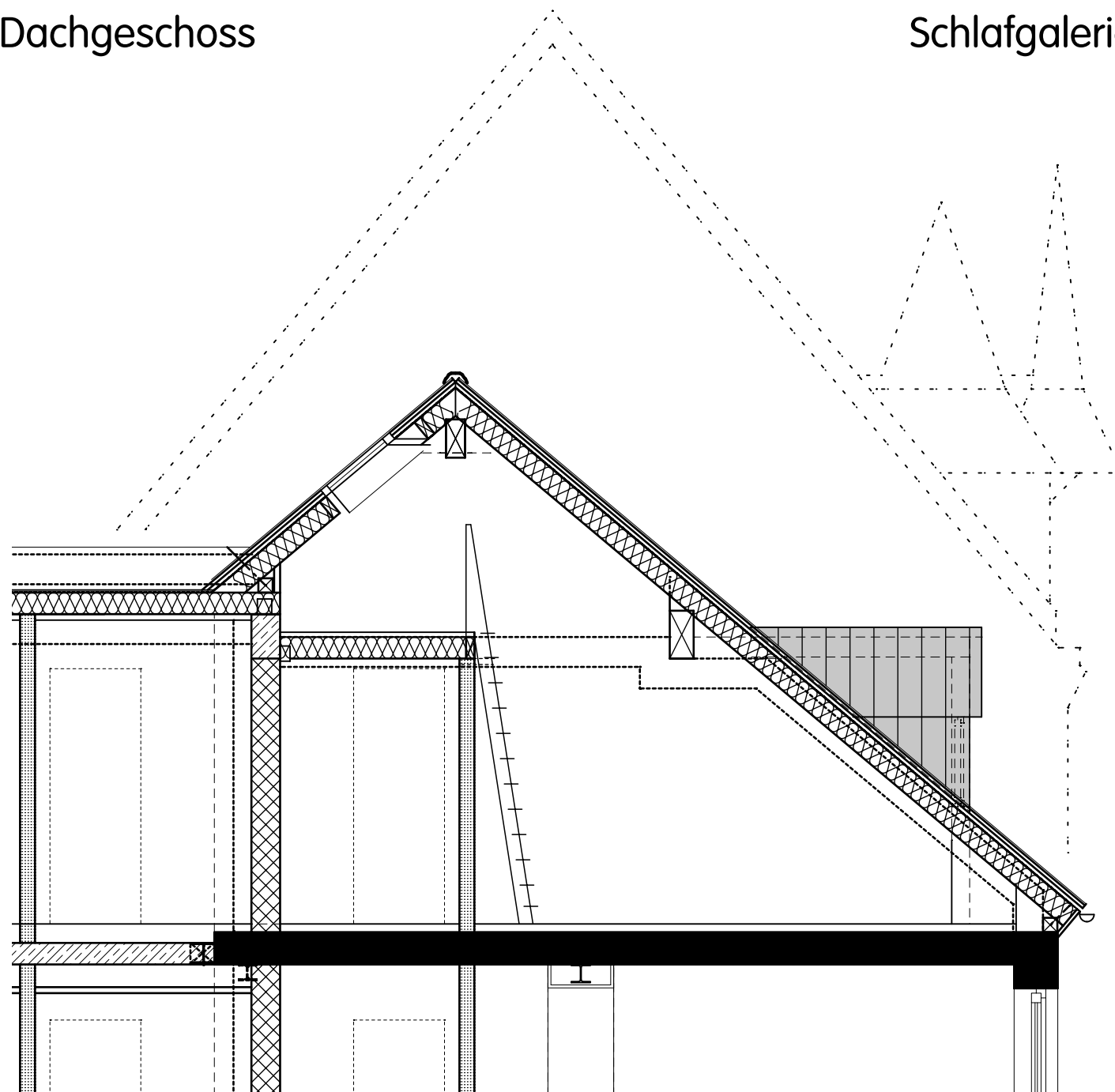
Schnitt
